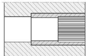
INSTALLAZIONE STANDARD
